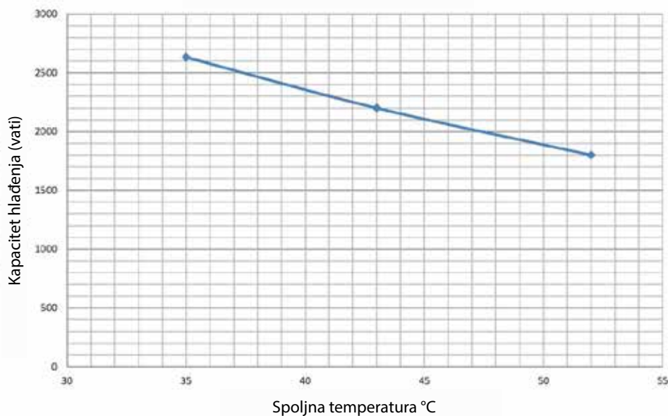
Test rashladne moći uređaja WZ-25 & WZ-25 EC sobna temperatura 27 °C
