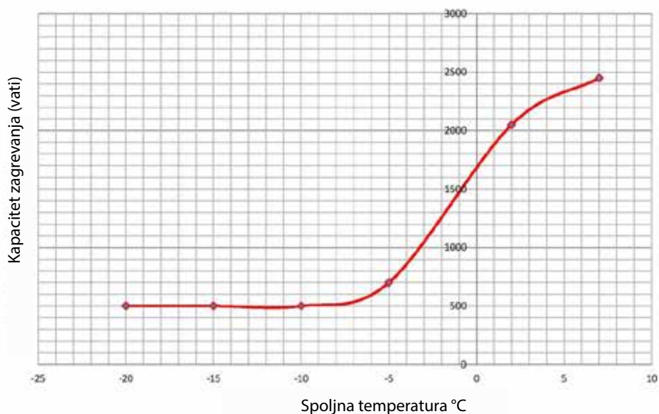
Test moći zagrevanja uređaja WZ-25 & WZ-25 EC sobna temperatura 20 °C
